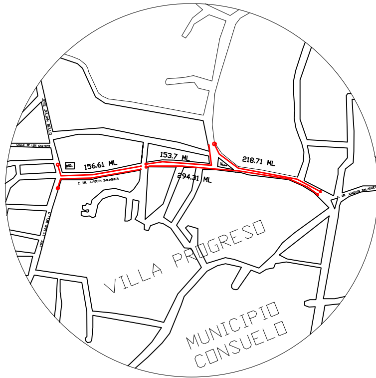
PLANO DE LOCALIZACION 975934ML DE ACERAS Y CONTENES
